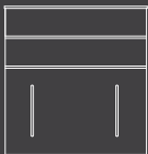
PIP - D128 1129W x 1701H x 407D
